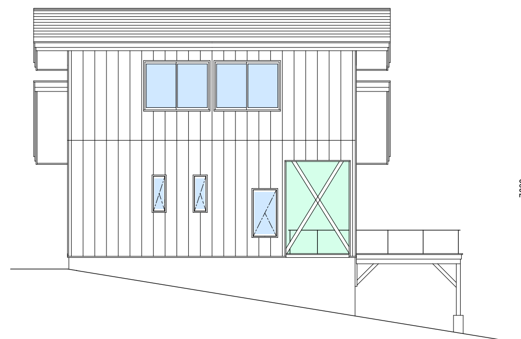
南立面図 S=1/100
